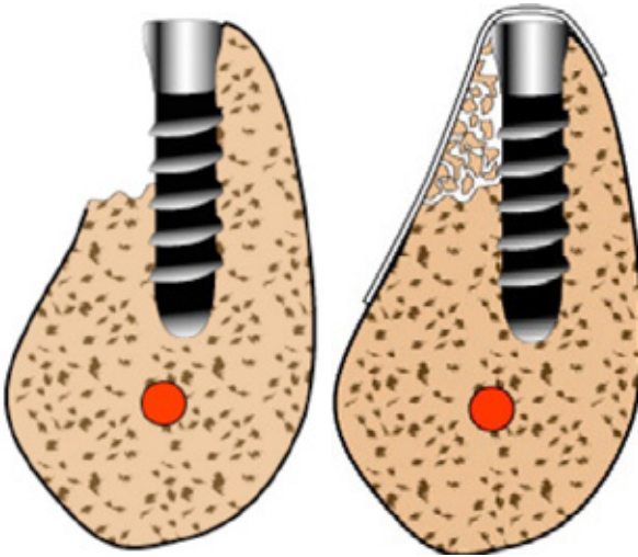
Figuur 1. Links het implantaat met ontbrekend bot en rechts met nieuw (kunst)bot met daaroverheen een membraan. Dit is een dun vliesje dat het aangebrachte bot scheidt van het tandvles. De grijze stip geeft de plaats van de zenuw aan (in dit geval de onderkaak).
